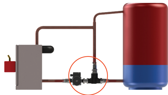
Laddomat 11 wird zwischen Kessel und Pufferspeicher platziert
